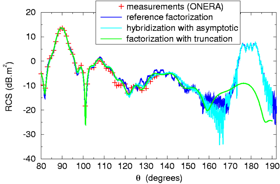
Figure 2 : RCS of the channel mock-up as a function of \theta for 7 GHz SER de la maquette du conduit en fonction de \theta pour 7 GHz
