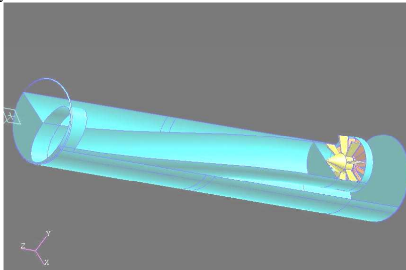
Figure 1 : Perspective of the channel mock-up Perspective de la maquette du conduit
