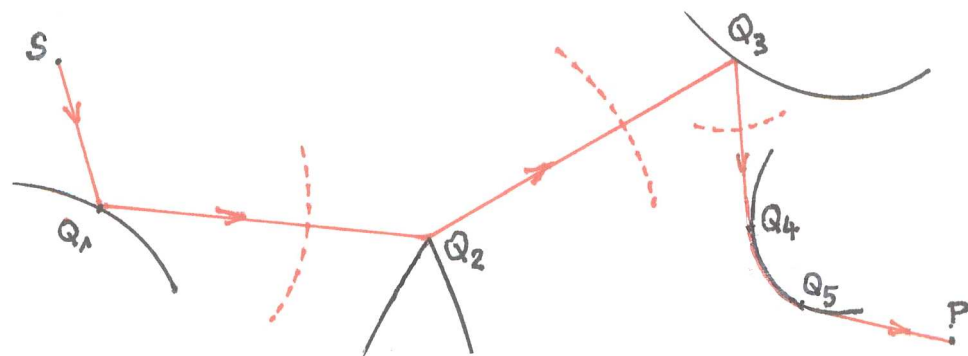
Figure 3 : Chain of interactions comprising reflections, edge diffractions and creeping waves Chaîne d'interactions comprenant des réflexions, des diffractions et des ondes rampantes
