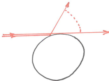
Figure 4 : Divergence of the reflected rays near the shadow boundary Divergence des rayons réfléchis près de la frontière d'ombre
